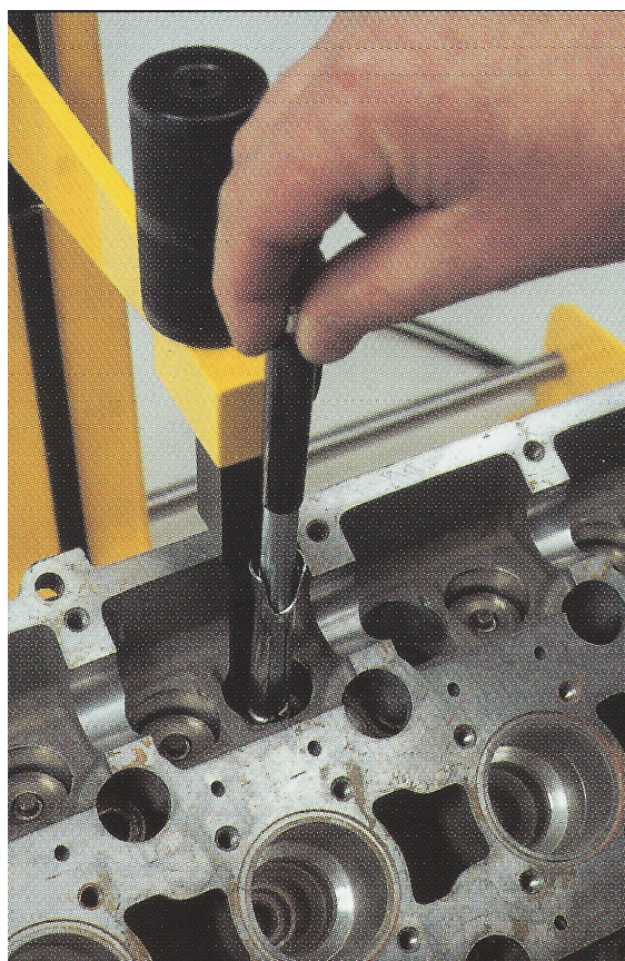
Installazione dei semiconi rapida e facile con gli installatori automatici, grazie al disegno aperto verticalmente dei premimolla..
